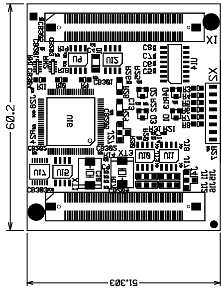
PHYTEC Messtechnik GmbH 1214.0 - PHYCORE-XC161
