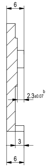
Schnitt A-A
