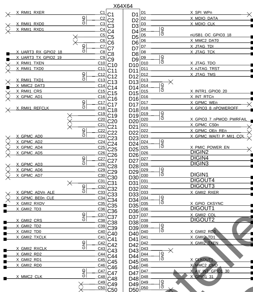
Optional Connector
