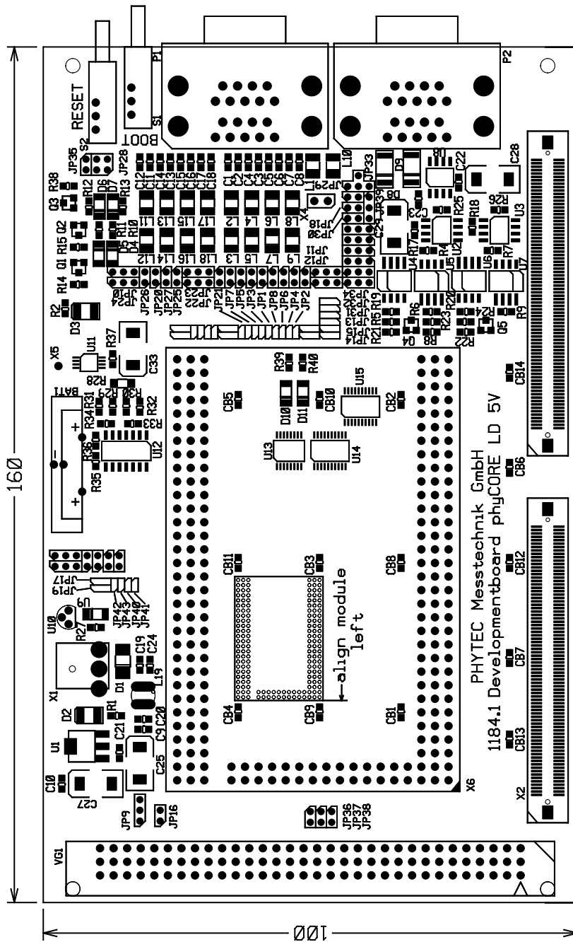
PHYTEC Messtechnik GmbH 1184.1 - Devboard phyCORE LD 5V
